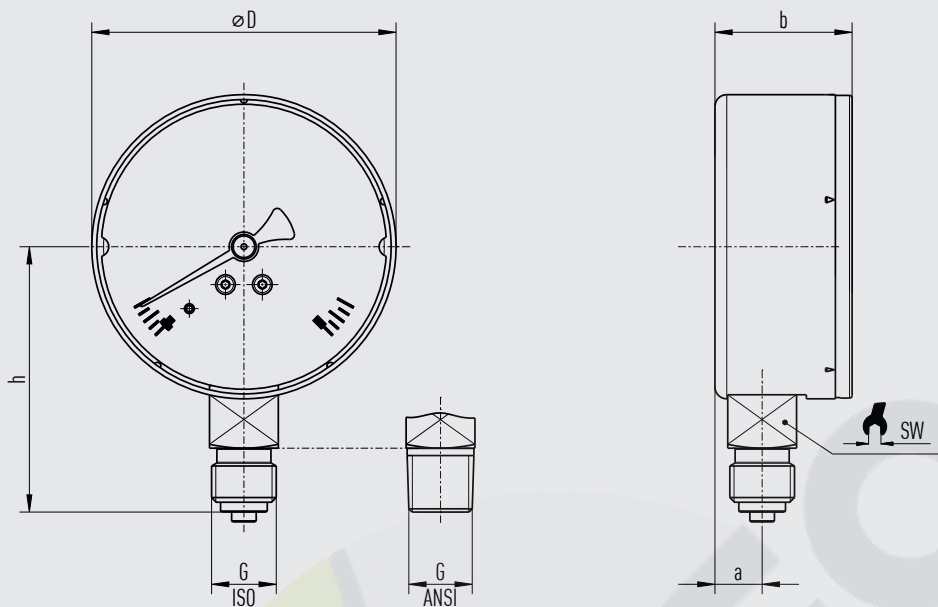
Modelo 131.11, conexión radial inferior
