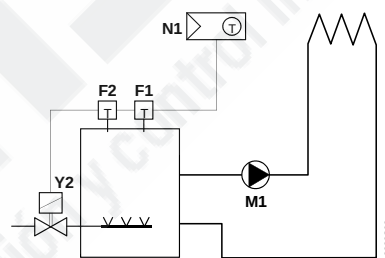
Controlador de temperatura ambiente con control directo de caldera de pie con quemador de gas
