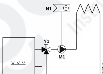
Controlador de temperatura ambiente con control directo de una bomba del circuito de calefacción (precontrol mediante válvula mezcladora manual)
