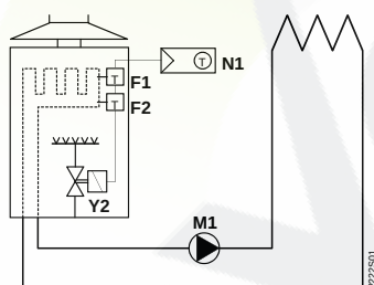
Controlador de temperatura ambiente con control directo de caldera mural con quemador de gas
