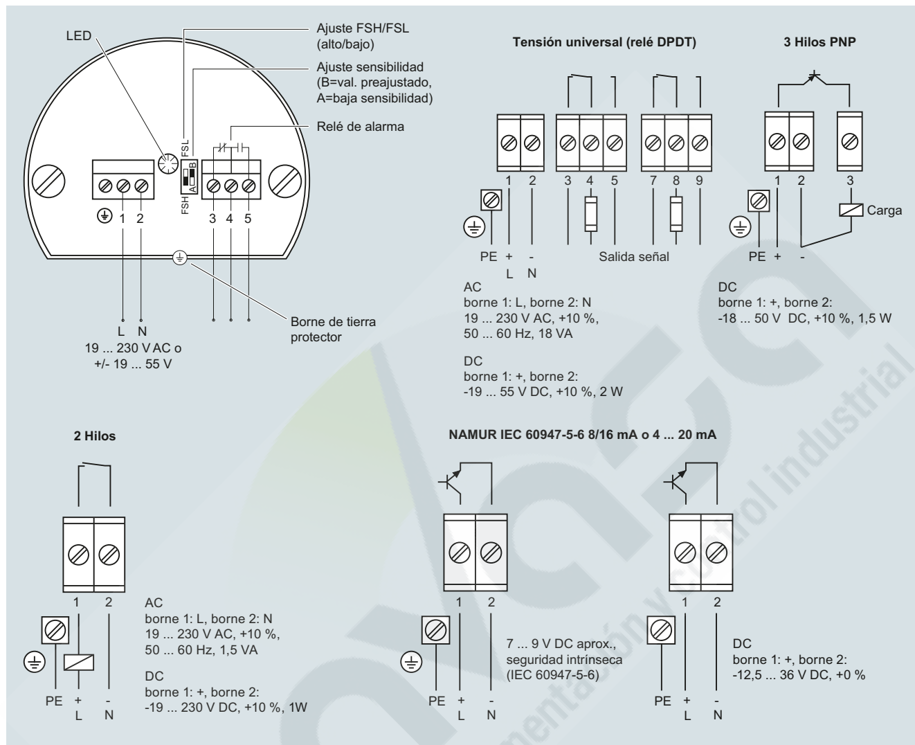
Conexiones SITRANS LVS200
