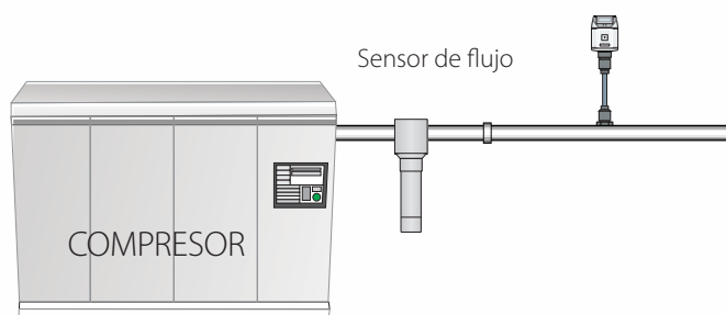
Medición de caudal generado por el compresor y cálculo FAD
