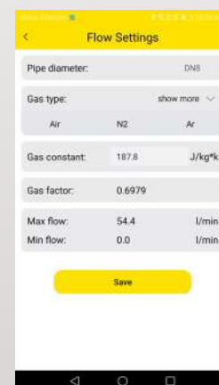
Configuración de flujo de un sensor
