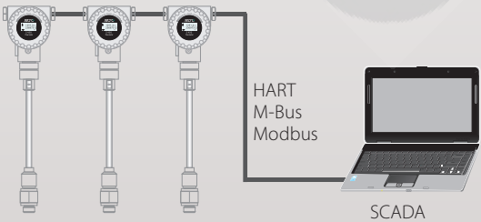
Comunicación industrial a través de Modbus, M-Bus, HART
