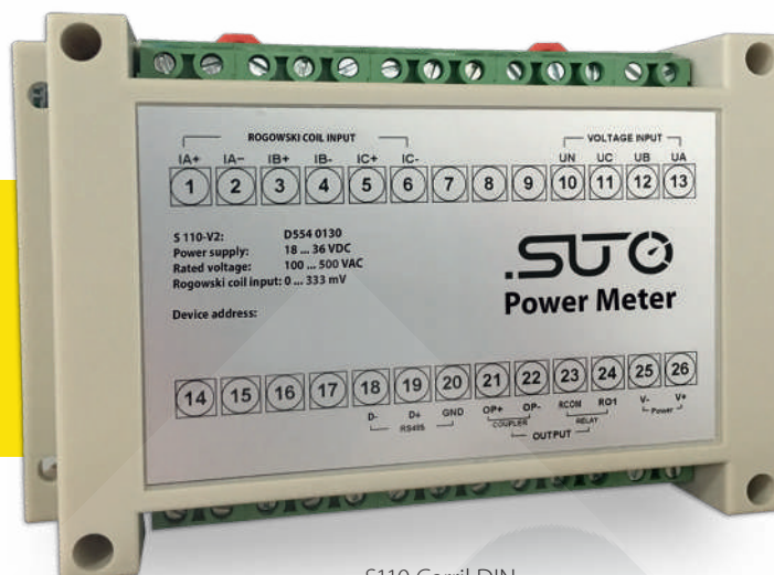
S110 Carril DIN
