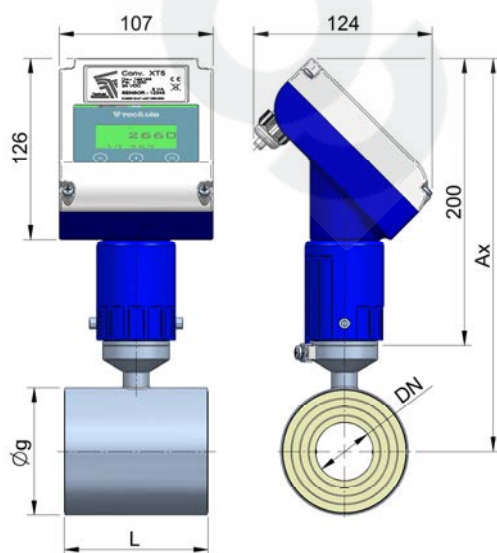
Convertidor XT5 montaje compacto
