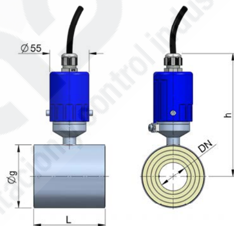
Convertidor montaje remoto
