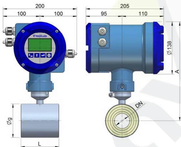
Convertidor XT5 montaje compacto
