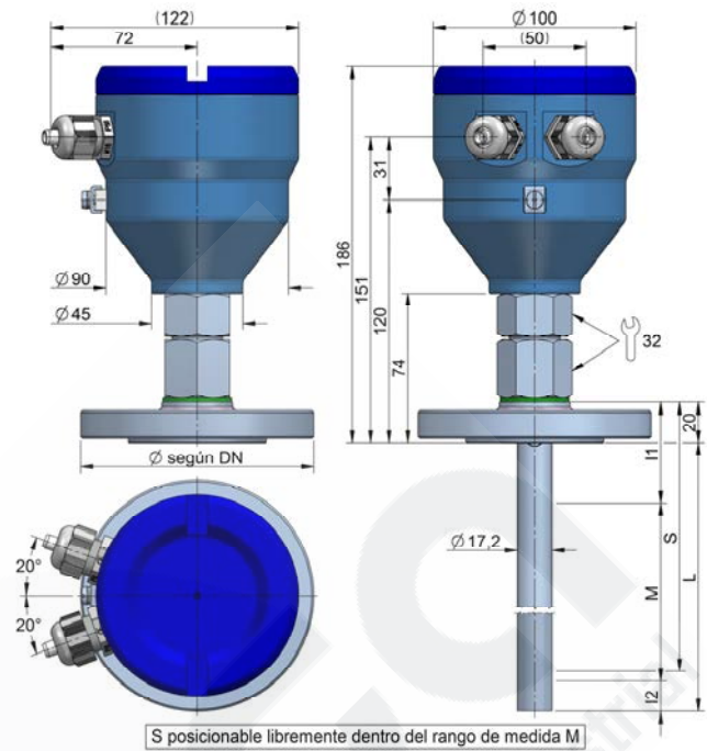
Sonda coaxial, conexión brida
