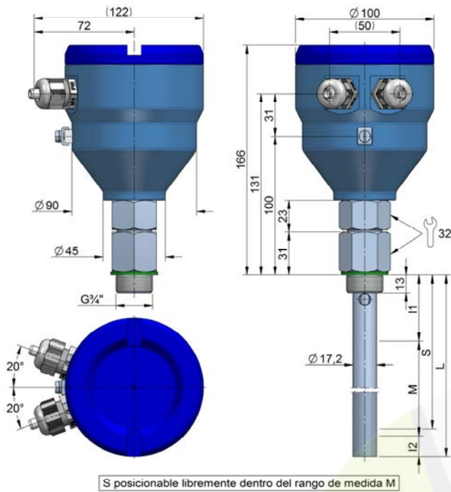
Sonda coaxial, conexión roscada
