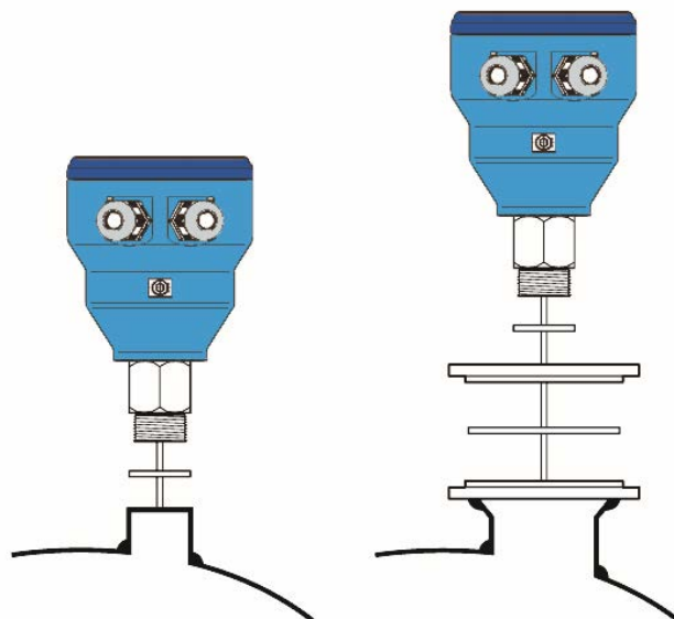
Instalación estándar transmisor LTDR
