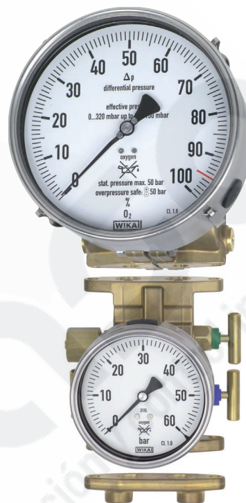
Fig. superior: Manómetro de presión diferencial modelo 712.15.160
