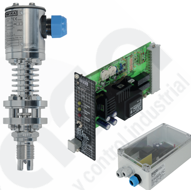
Fig. izquierda: Modelo OLS-H versión de alta presión Fig. central: Modelo OSA-S, tarjeta enchufable de 19" Fig. a la derecha: Modelo OSA-S, envoltorio de montaje de policarbonato
