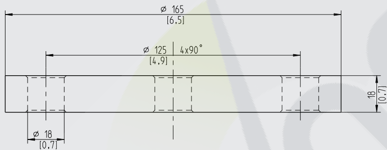
Brida DN 50, forma B según EN 1092-1 (DIN 2527), PN 16
