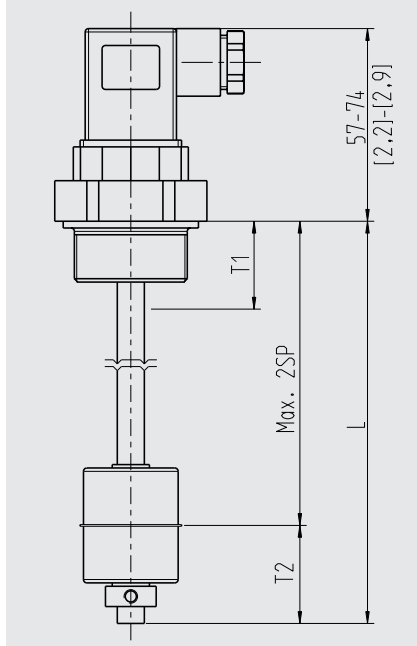
con conector angular forma A
