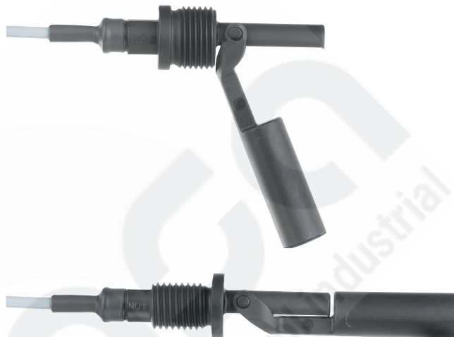
Fig. superior: Modelo RLS-8000 con G 1/2, montaje desde el exterior
