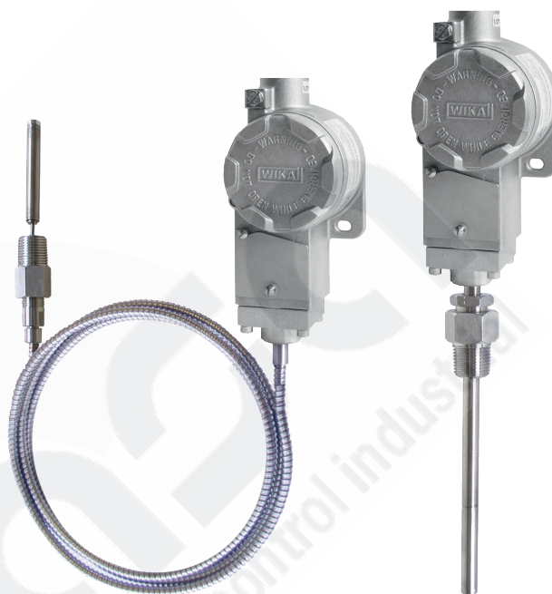
Fig. izquierda: Montaje con capilar Fig. derecha: Montaje directo
