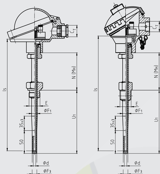
Rosca cilíndrica
