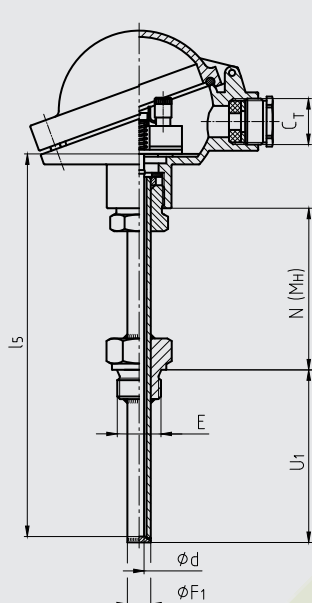
Rosca cilíndrica
