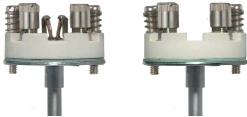
Fig. izquierda: Versión estándar Fig. derecha: Versión con lengüetas de soldadura encapsuladas (opcional)
