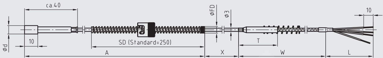
Punta del sensor plana
