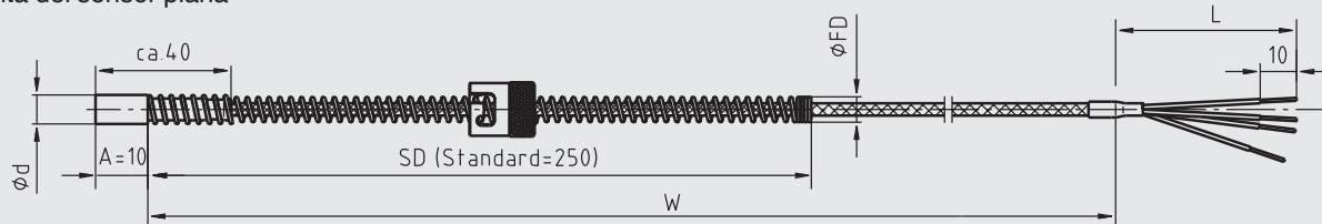
Punta del sensor plana
