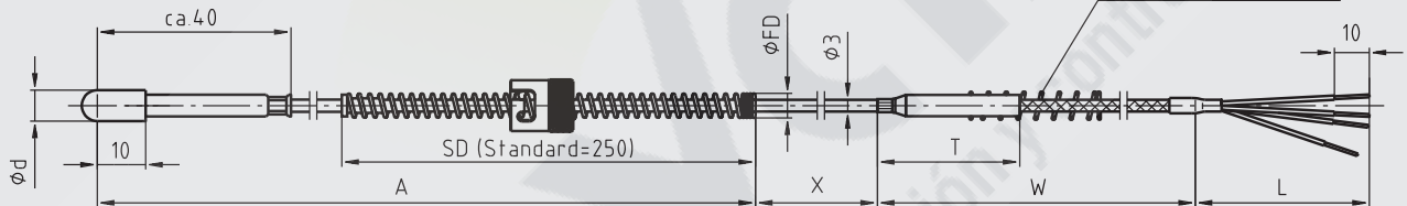
Punta del sensor redonda
