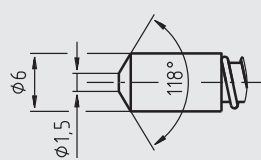
Punta del sensor redonda
