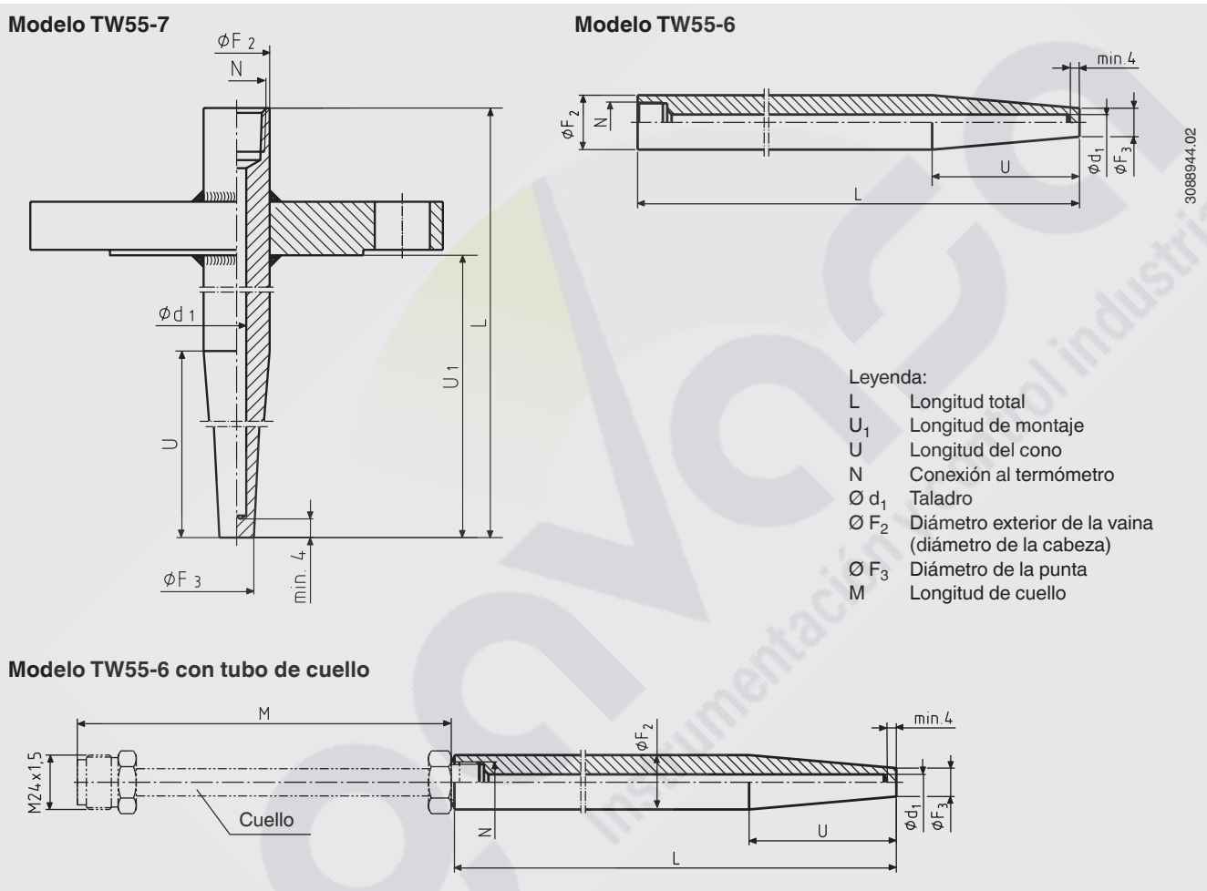
Longitudes estándares modelo TW55-7
