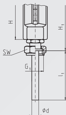
Forma de conexión 3, tuerca loca (sólo con tamaño nominal 200)
