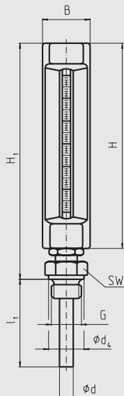
Forma de conexión E, racor roscado
