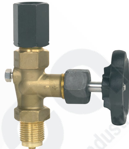
Válvula de cierre según DIN 16270, Racor de sujeción hembra /macho G 1/2, PN 250
